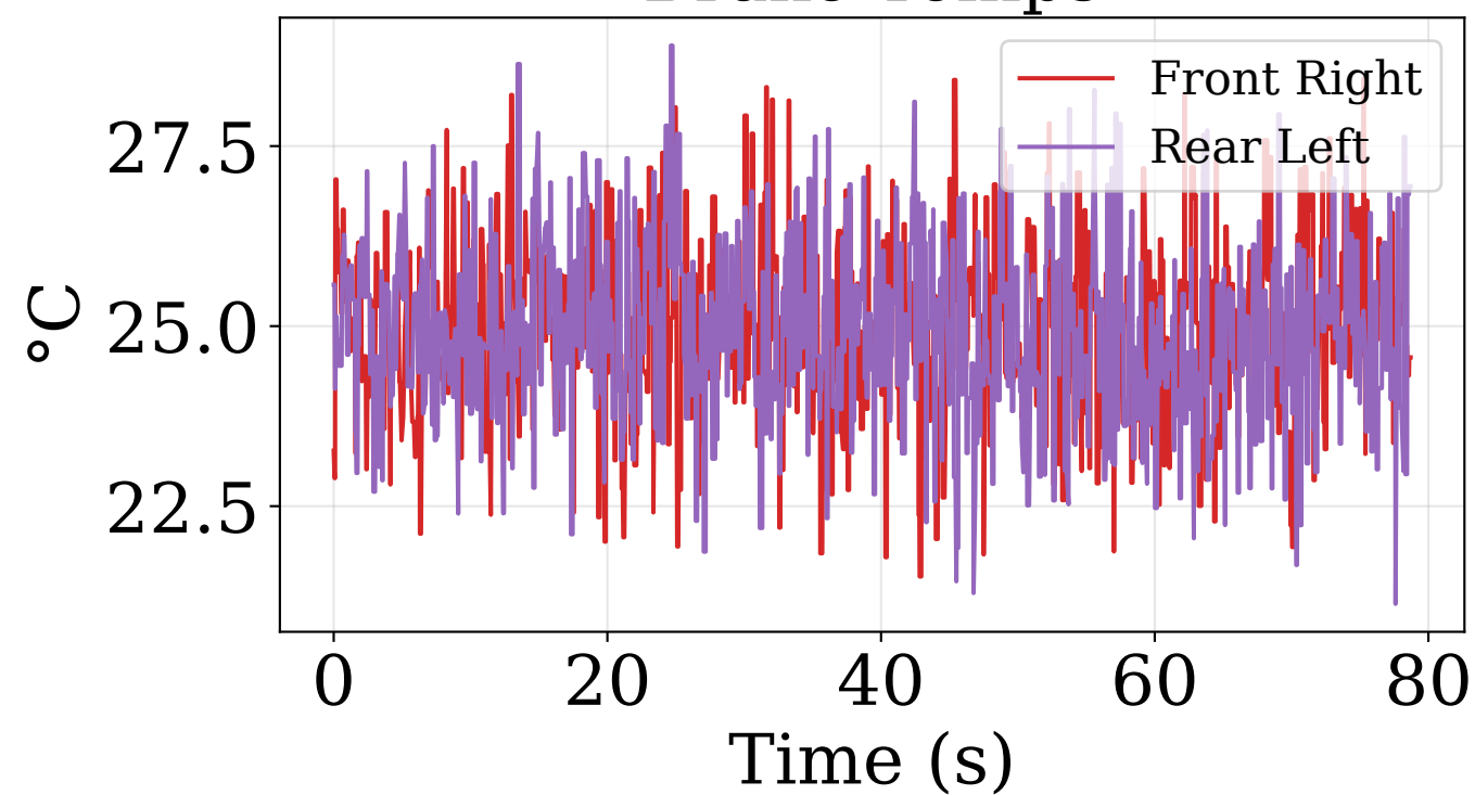
Brake Temps
