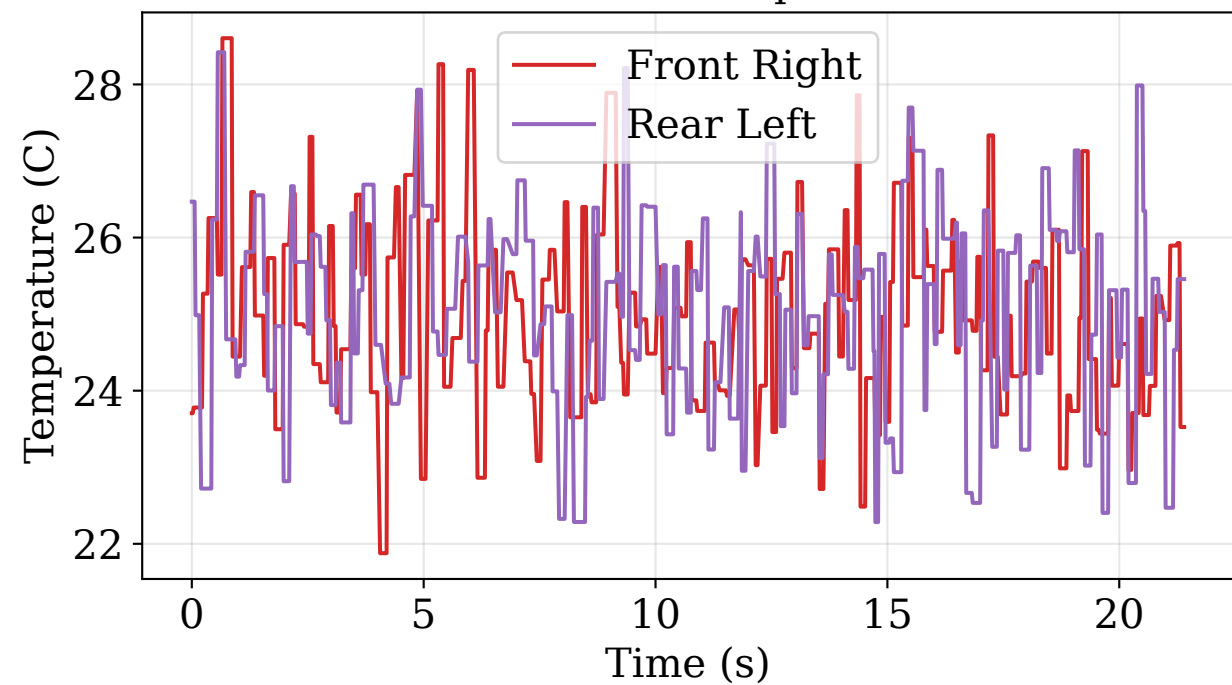
Brake Temps
