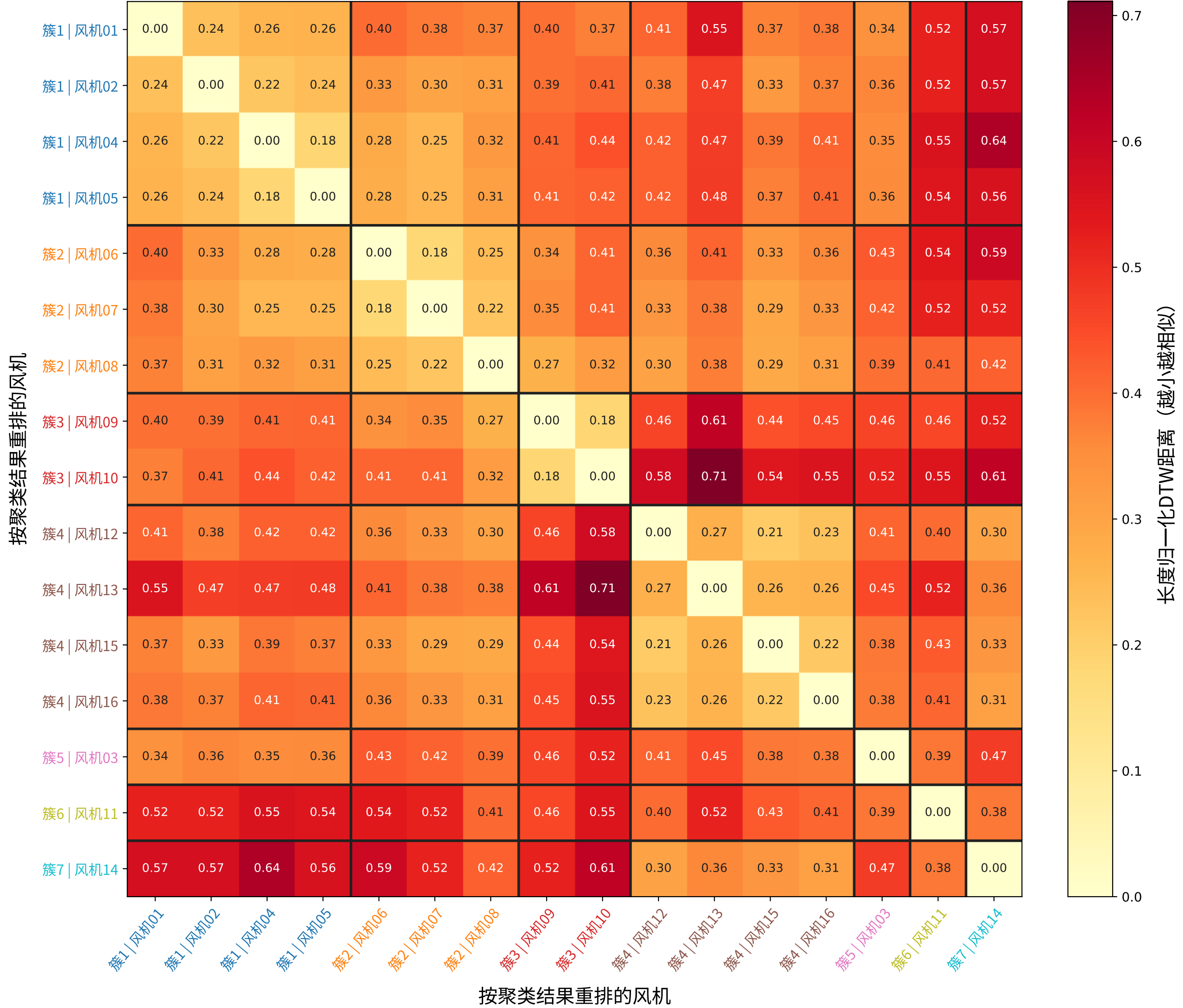
2026年5月24日16台风机DTW聚类热力图（7簇） 完全链接层次聚类 | 高相似距离阈值 < 0.30 | 每台8640个原始10秒点
