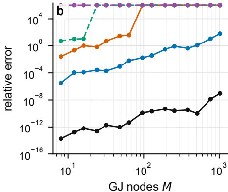
GJ-II: raw quotient precision
