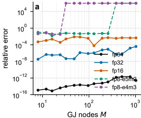
GJ-I: raw quotient precision
