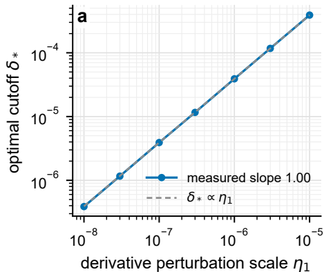
Type-I optimum
