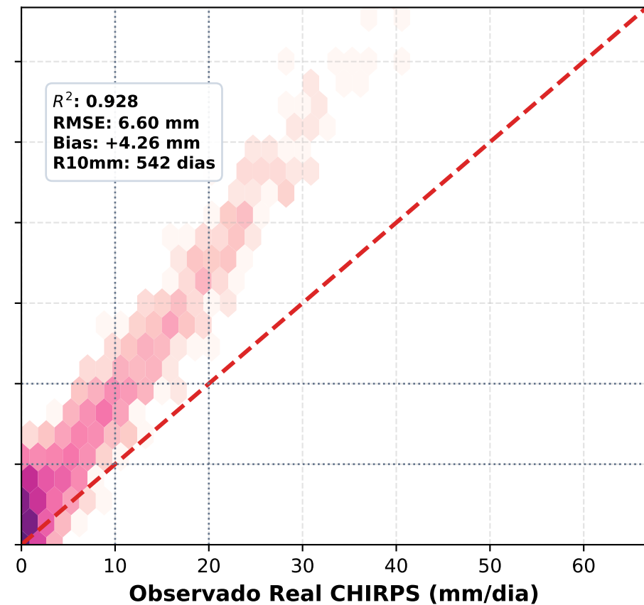
EQM (2012)
