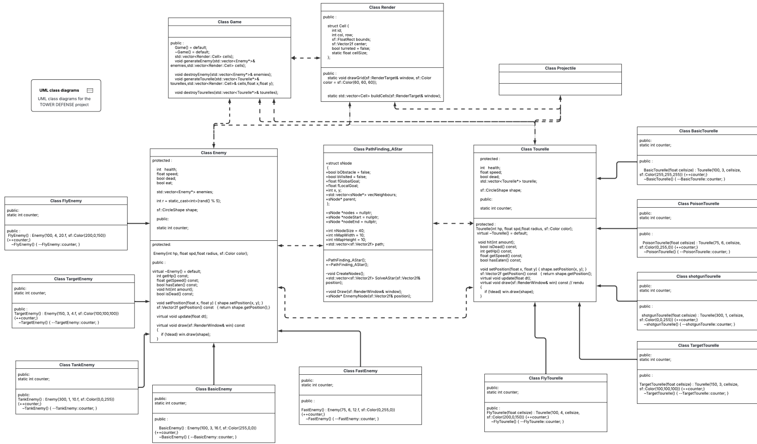
Figure 3: Diagramme de classes du projet.
