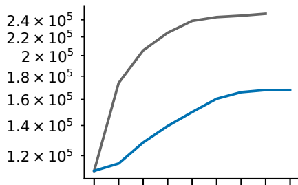
LiH, HF
