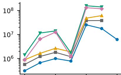
LiH 3.0 Å
