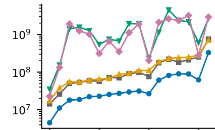
H_2O eq
