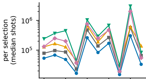
H_4 1.0 Å
