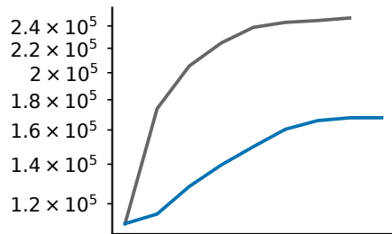
LiH, HF
