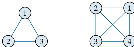
Vollstndiger Graph K_3 Vollstndiger Graph K_4
