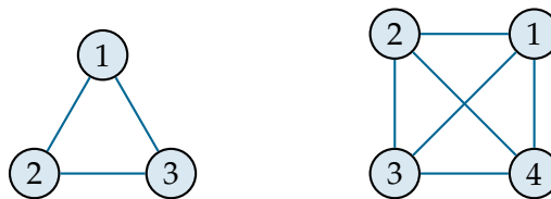
Vollständiger Graph K_3 Vollständiger Graph K_4
