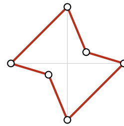
Oktaeder
