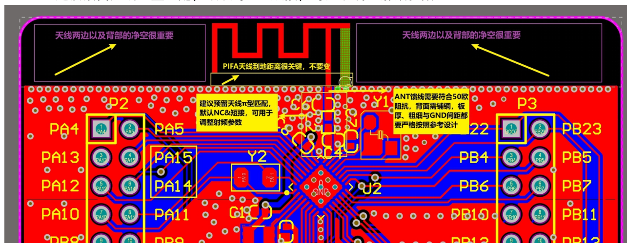
图 1. 天线设计注意事项
