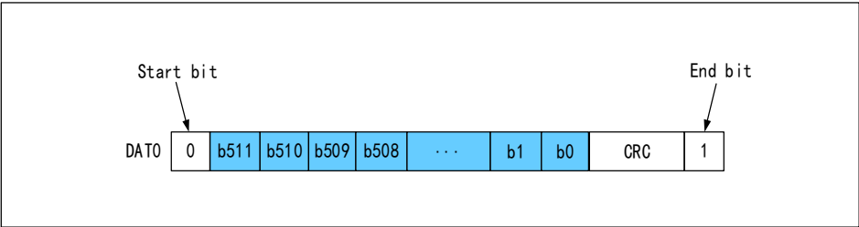
图 24-11 SD 卡单总线数据传输一个 512 位字的格式
