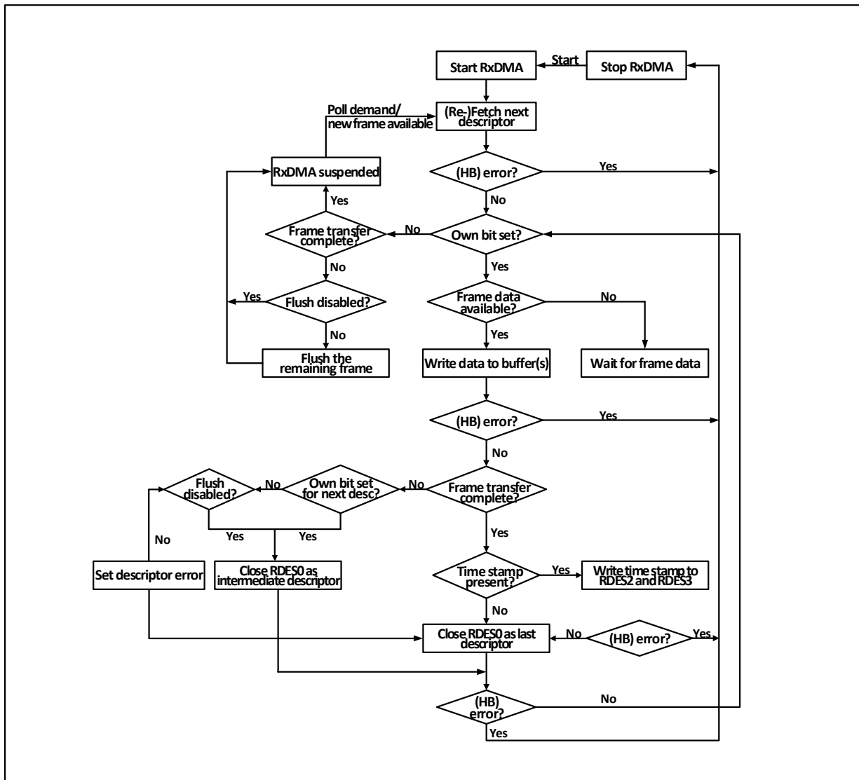
图 29-5 接收流程
