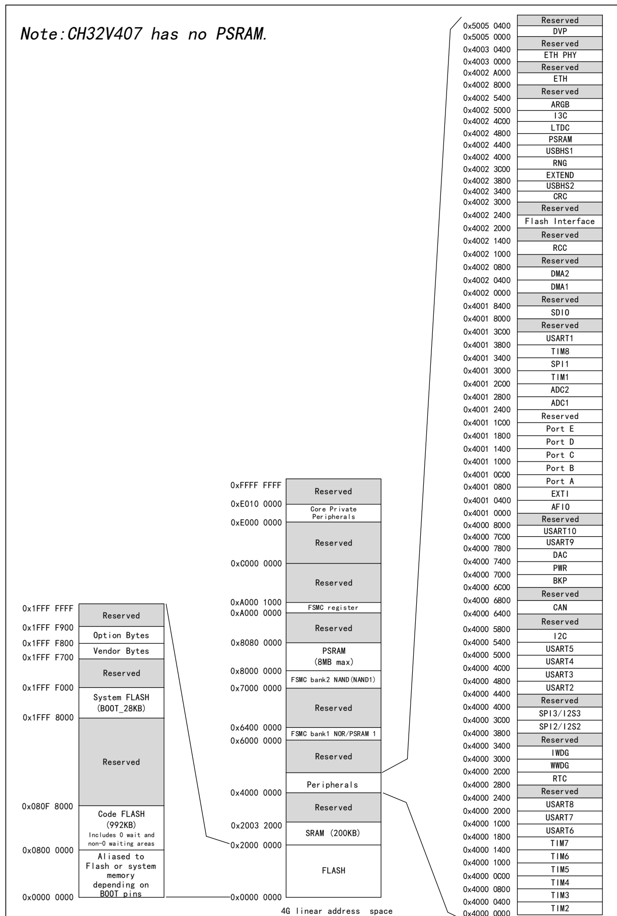
图 1-2 存储映像
