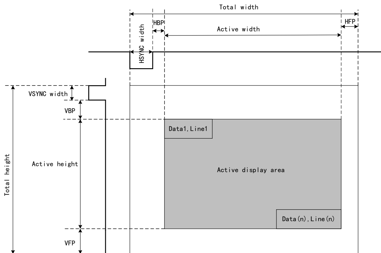
图 27-2 LTDC 同步时序
