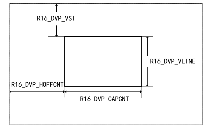
图 23-5 裁剪窗口的坐标和大小
