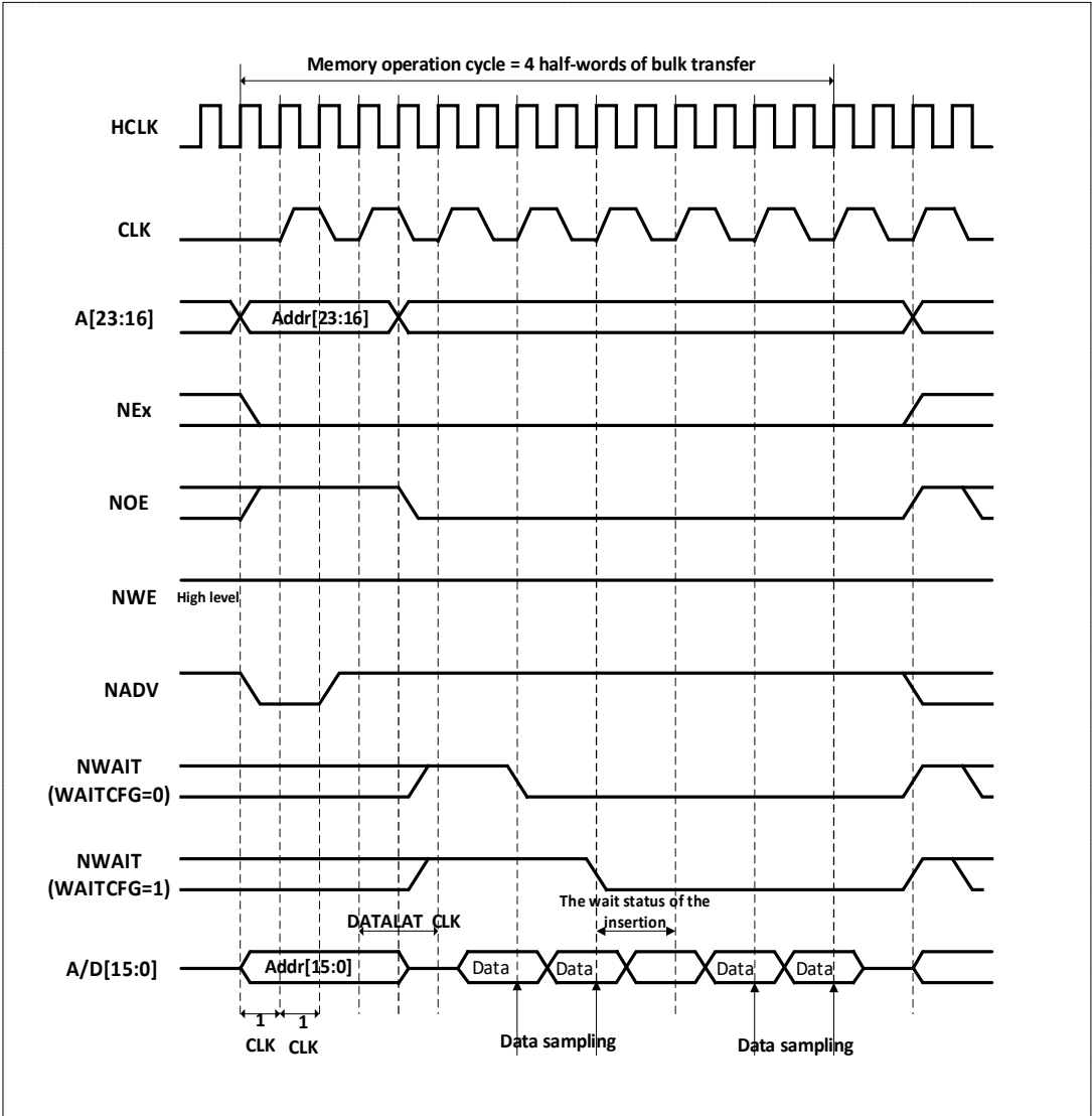
图 26-13 同步总线复用读操作（复用）
