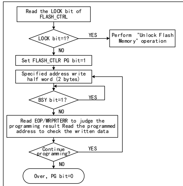
图 32-1 FLASH 编程
