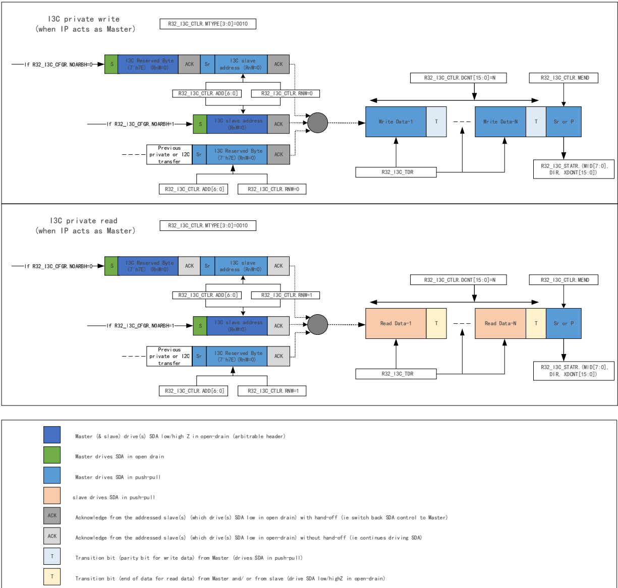
图 19-5 I3C 私有读/写消息（作为主设备）
