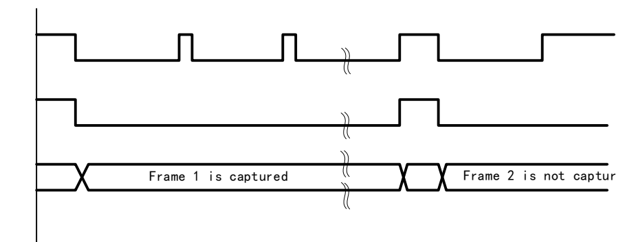
图 23-3 快照模式下的单帧捕获波形
