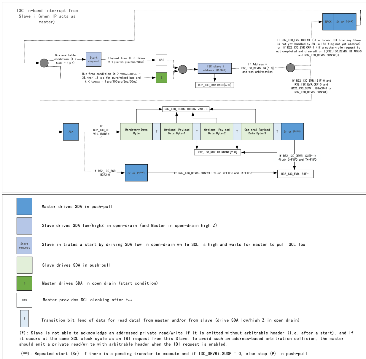
图 19-7 I3C IBI 传输（作为主设备）
