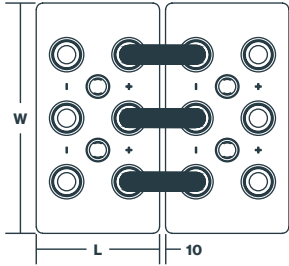
14 OPzS-ET1750 a 18 OPzS-ET2250
