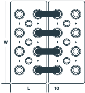
19 OPzS-ET2375 a 26 OPzS-ET3250
