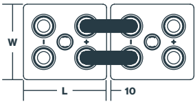
8 OPzS-ET800 a 13 OPzS-ET1625
