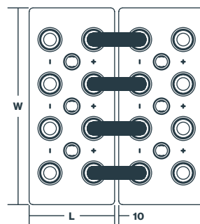
19 OPzV-ET 3135SOLAR a 26 OPzV-ET 4250SOLAR
