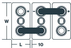
2 OPzV-ET 140SOLAR a 7 OPzV-ET 1050SOLAR
