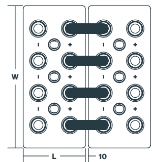
19 OPzV-ET 2375 a 26 OPzV-ET 3250
