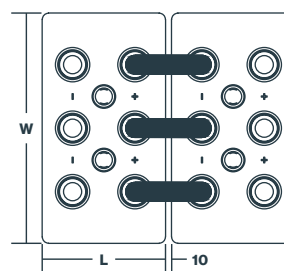
14 OPzV-ET 1750 a 18 OPzV-ET 2250
