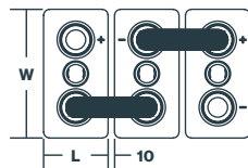
2 OPzV-ET 100 a 7 OPzV-ET 700
