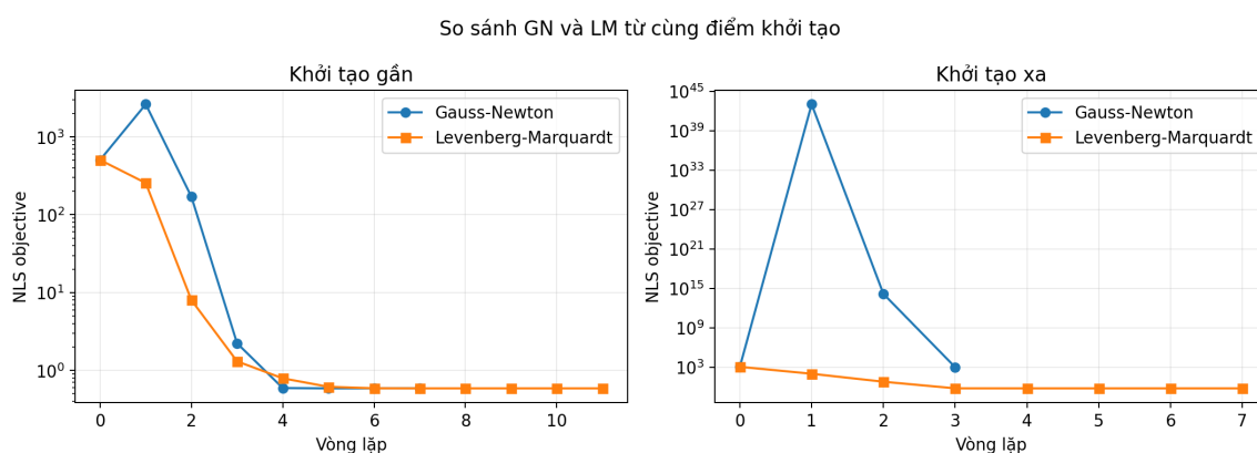
Hình 6.3: Lịch sử objective của Gauss–Newton và Levenberg–Marquardt với hai cách khởi tạo.
