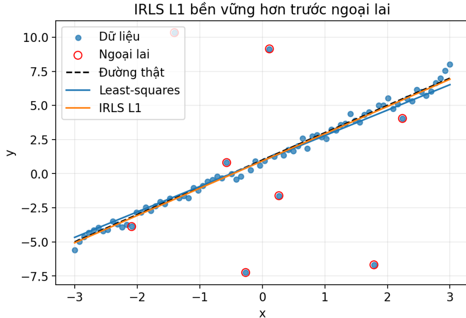
Hình 6.4: So sánh least-squares và IRLS L^1 trên dữ liệu có ngoại lai.
