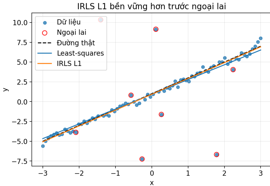
Hình 6.4: So sánh bình phương tối thiểu và IRLS L^1 trên dữ liệu có ngoại lai.
