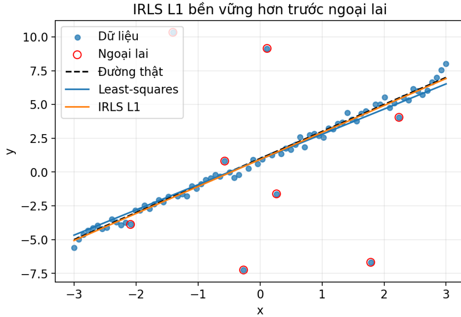
Hình 6.4: So sánh least-squares và IRLS L^1 trên dữ liệu có ngoại lai.
