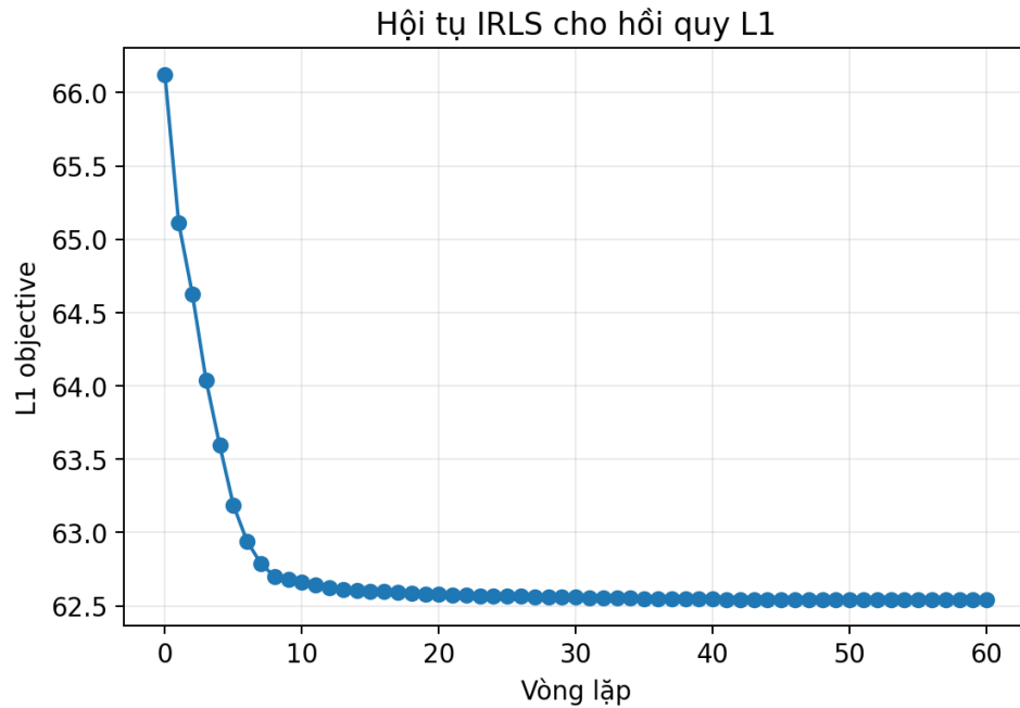
Hình 6.5: Sự thay đổi của objective L^1 trong quá trình lặp IRLS.
