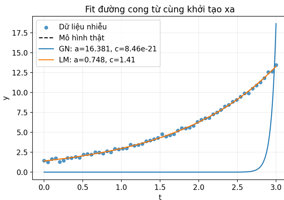
Hình 6.2: Kết quả fit đường cong của hai phương pháp từ cùng một khởi tạo xa.
