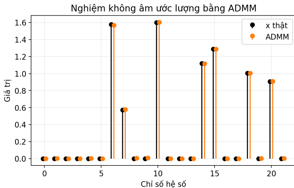
Hình 6.10: So sánh nghiệm không âm do ADMM ước lượng với vector hệ số thật.
