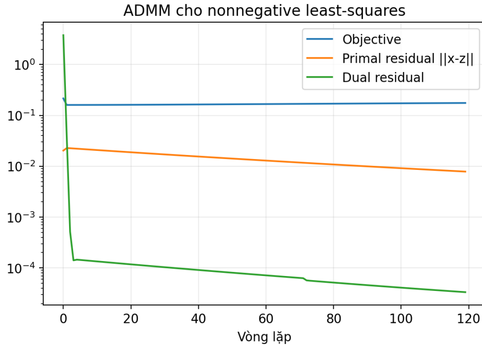
Hình 6.9: Objective, primal residual và dual residual của ADMM cho NNLS.
