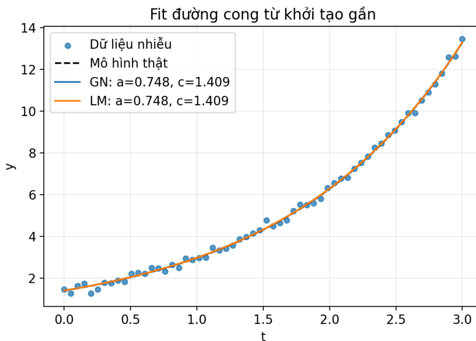
Hình 6.1: Kết quả fit đường cong của Gauss–Newton và Levenberg–Marquardt từ khởi tạo gần.
