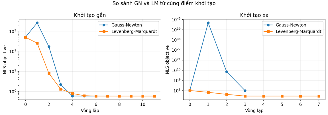
Hình 6.3: Lịch sử objective của Gauss–Newton và Levenberg–Marquardt với hai cách khởi tạo.
