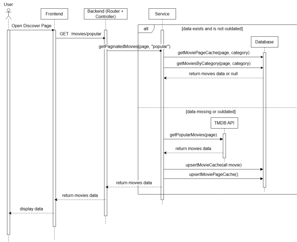
4.1 Adatfolyam diagram
