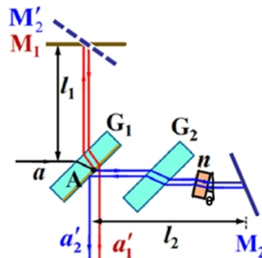
图 3.1.3.2 介质片旋转后的干涉示意图
