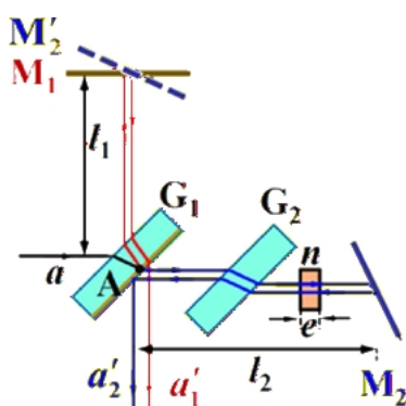
图 3.1.3.1 插入介质片后的干涉示意图
