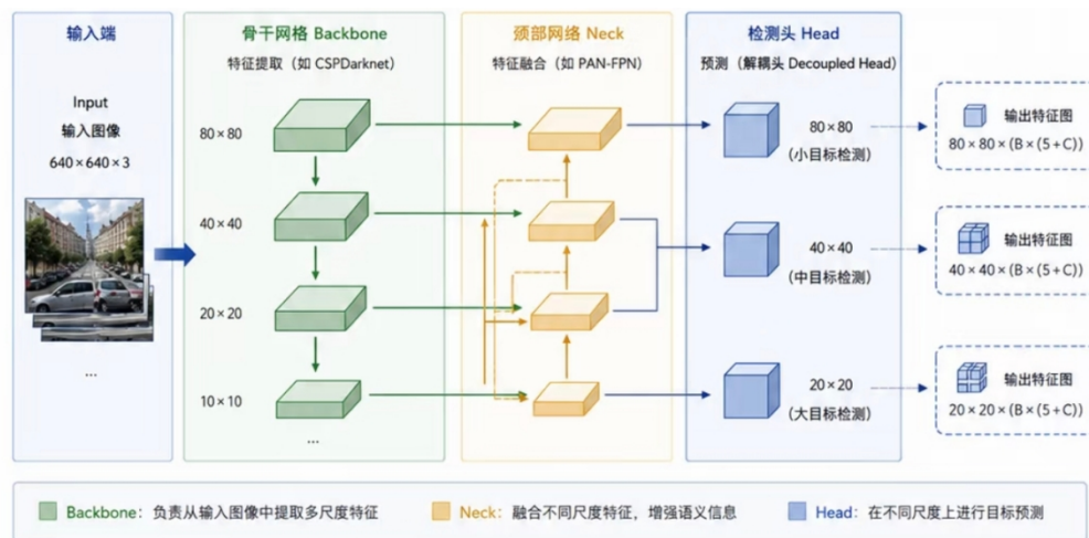
图 3.2.1.1 YOLOv8 结构框架图
