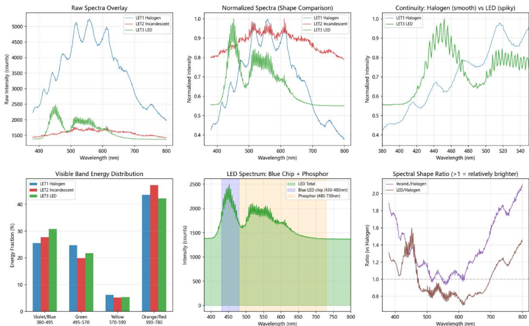
图 3.1.2.1 三类常见白光光源：卤素灯、白炽灯和 LED 灯的光谱分析
