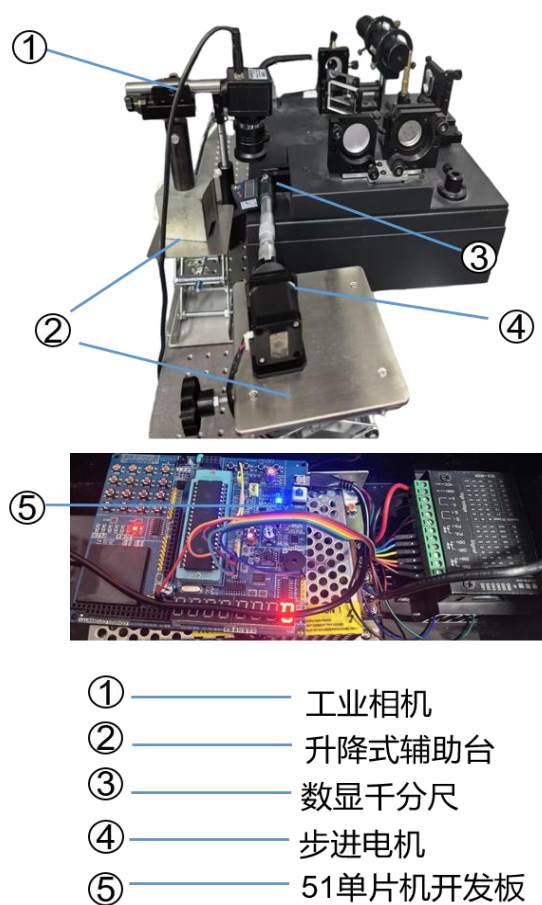
图 4.3.1 动静辅助调节系统图片
