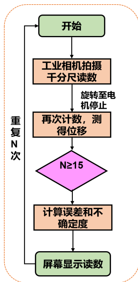
图 4.3.2 动静辅助调节系统工作流程
