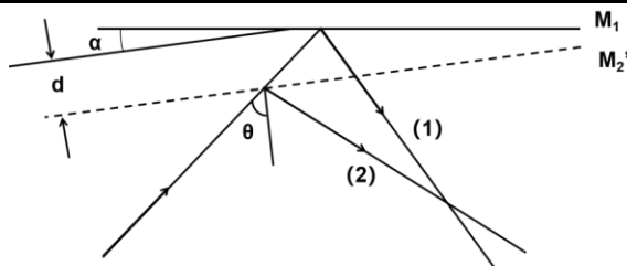
图 3.1.2 等厚干涉示意图
