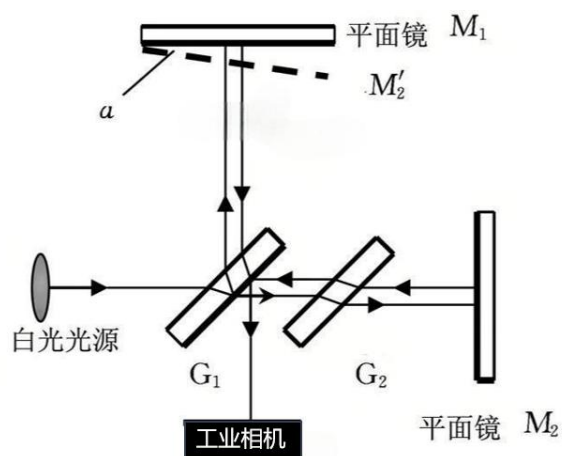
图 3.1.1 迈克尔逊白光干涉实验光路图
