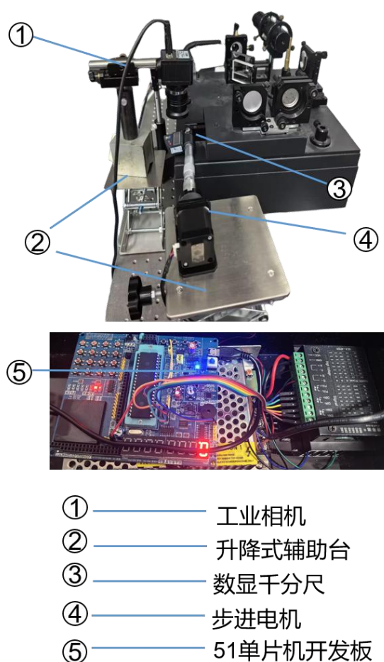
图 4.3.1 动静辅助调节系统图片
