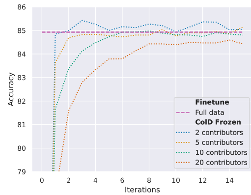
(d) Effect of Distributing
