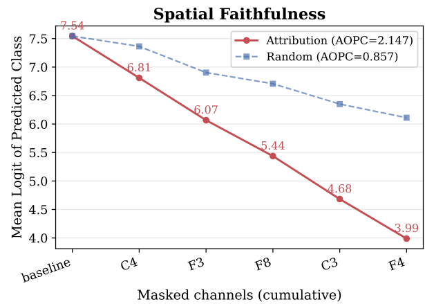
(d) Class 1 (MDD) – Spatial Faithfulness
