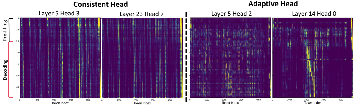
(b) Llama-3.1-8B
