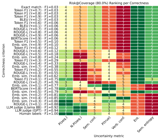
(a) Llama 3B
