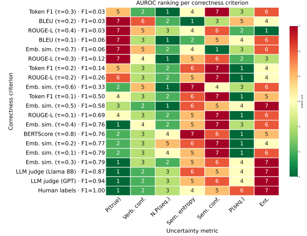
(b) Llama 8B, AmbigQA (ambiguous)
