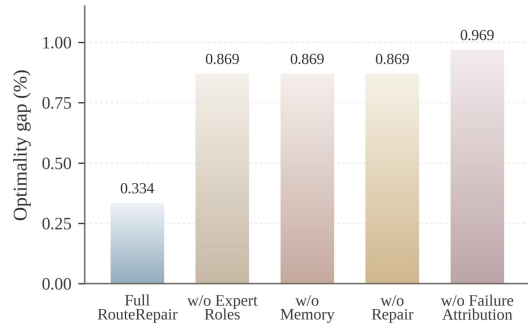
(b) TSP50
