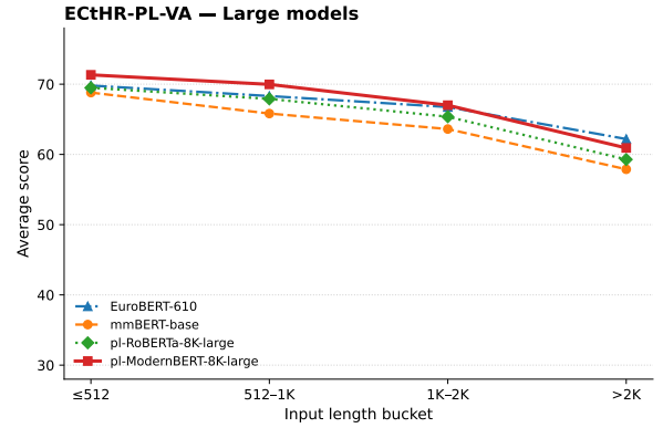
(d) ECTHR-PL-VA: Large models.
