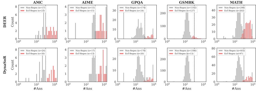
(d) QwQ-32B
