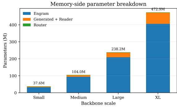
(b) Memory-side parameter scaling.
