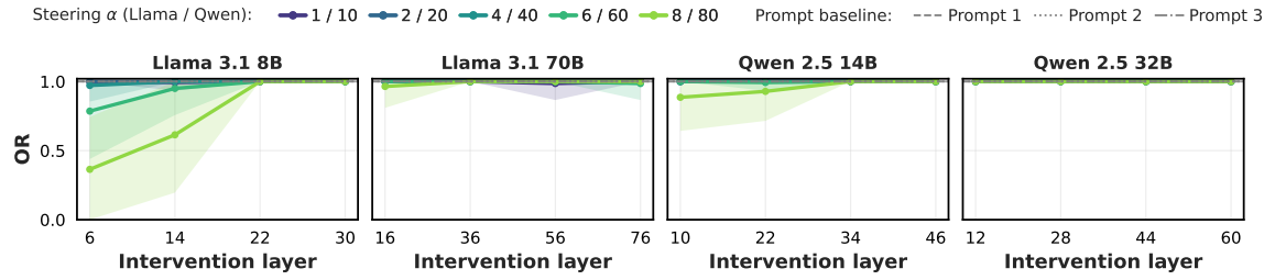
(b) Output Relevance (OR).
