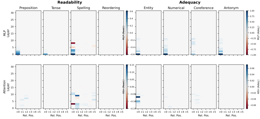
(a) Themis (Llama-3-8B)
