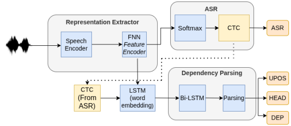
(a) Baseline Wav2tree (Pupier et al., 2024)
