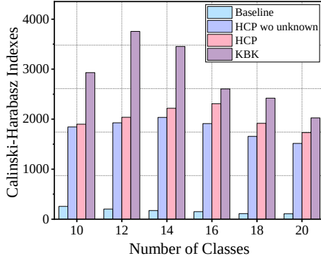
(a) Calinski-Harabasz indexes
