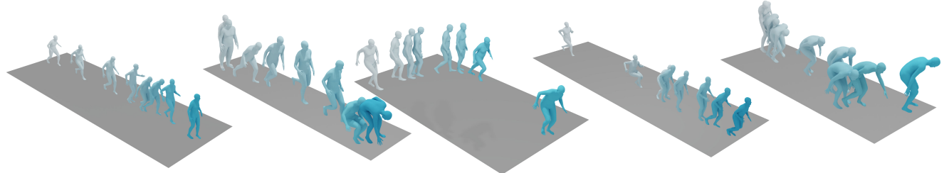
Ours
