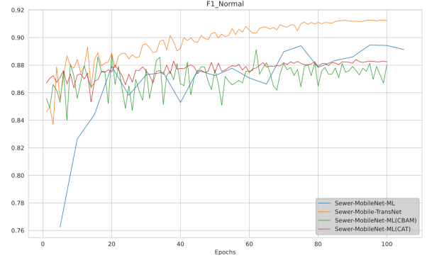
Fig. 10. F1 Score Curve Comparison
