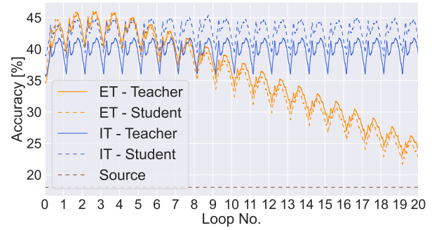
(d) RoTTA, ViT-B16
