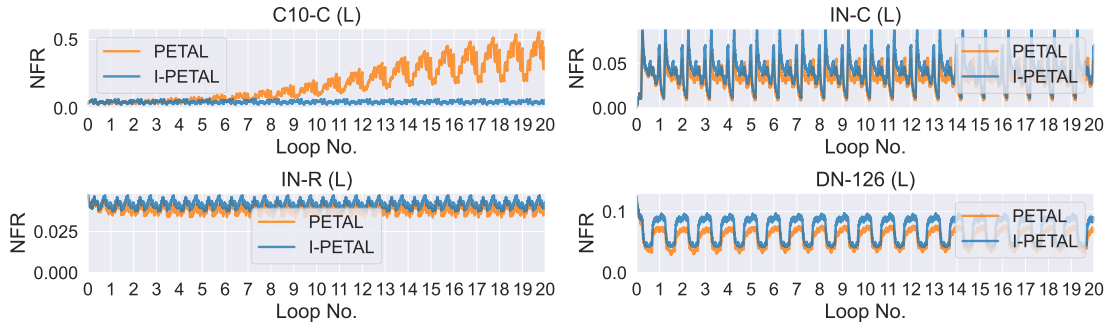
(d) PETAL
