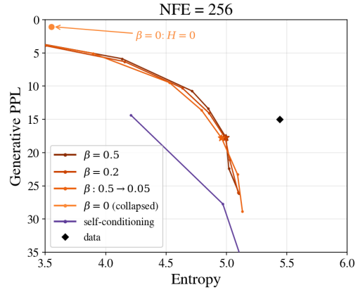
(d) Reinforce-DMD, NFE = 256
