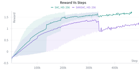
(d) Hidden dimension 256
