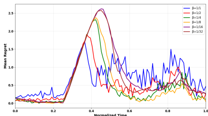
(g) Hartmann3
