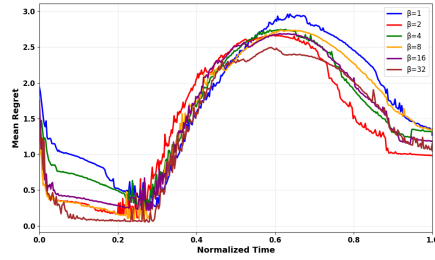
(h) Hartmann6
