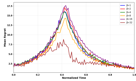
(d) Ackley
