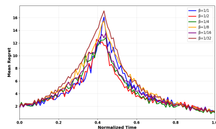
(d) Ackley
