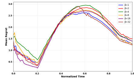
(h) Hartmann6
