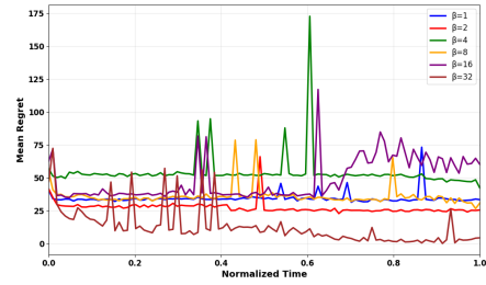
(f) Griewank
