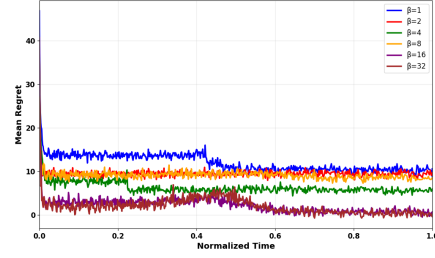
(f) Griewank
