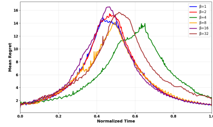
(d) Ackley
