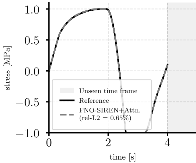
(e) Stress field till t8 (4 s)
