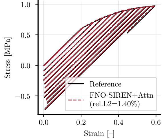
(d) FNO-SIREN+Attention
