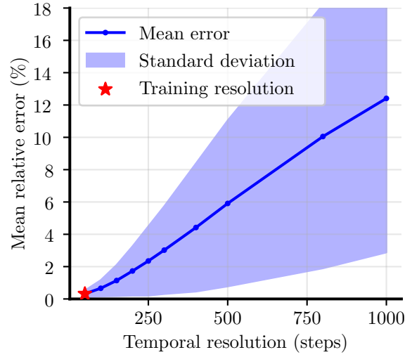
(d) RNN-GRU
