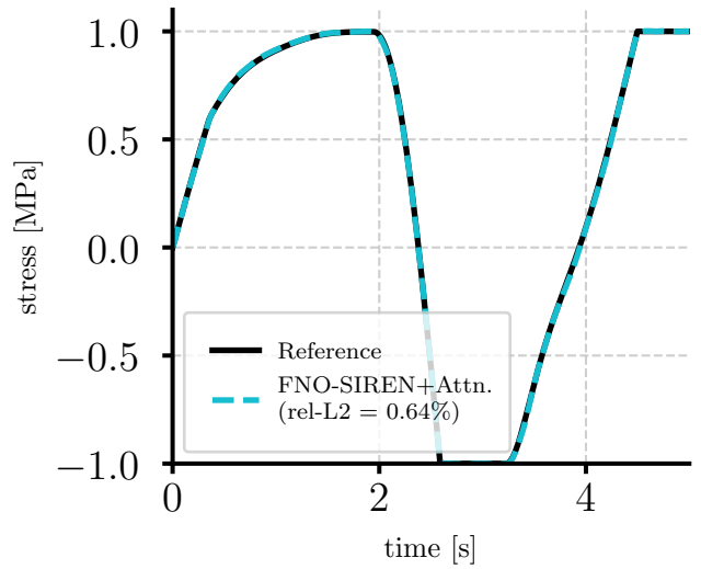
(f) Stress field till t10 (5 s)
