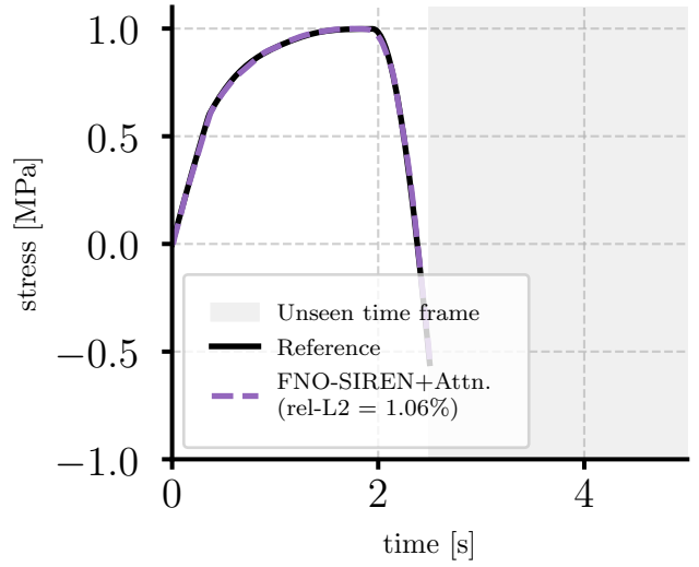
(d) Stress field till t5 (2.5 s)
