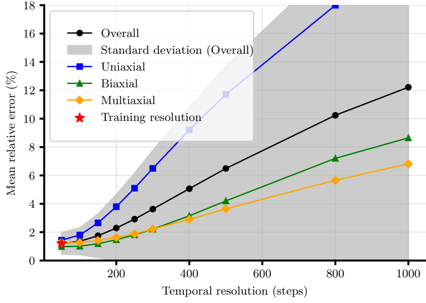
(a) RNN-GRU
