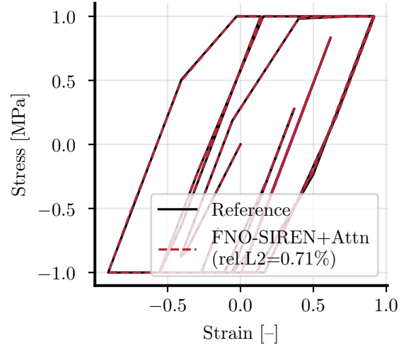
(d) FNO-SIREN+Attention
