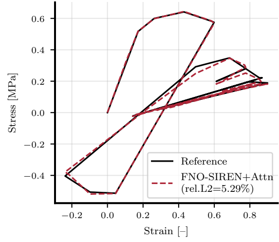
(d) FNO-SIREN+Attention
