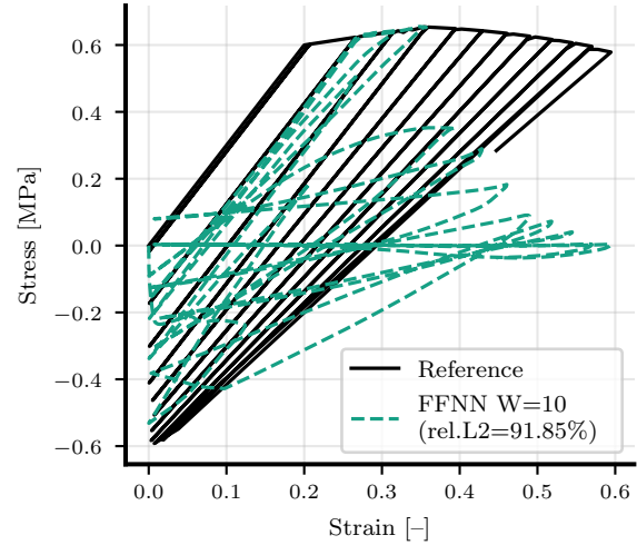
(b) FFNN(W = 10)
