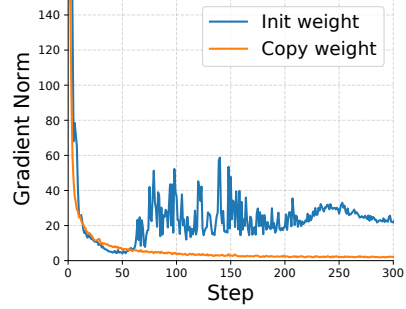
(b) Gradient norm.
