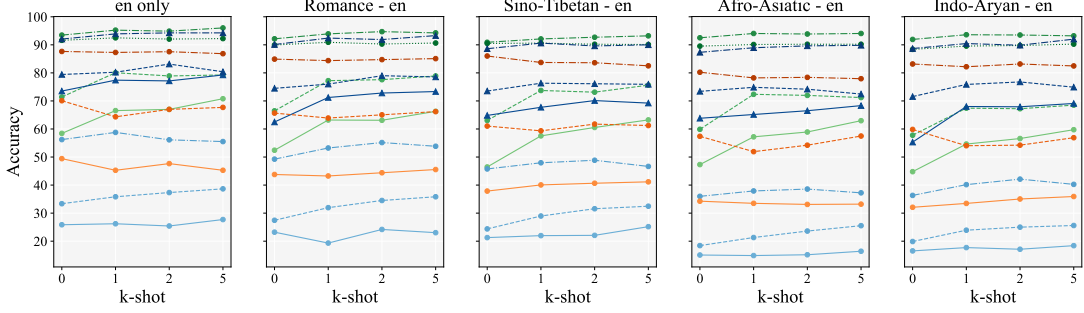
(b) CM-GSM8K
