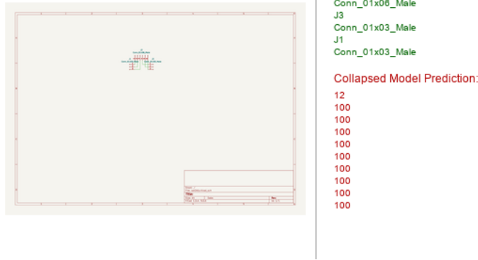
图 4: 旧模型 (V4, +Projector LoRA r = 16 ) 输出: 全部 50 个测试样本输出完全相同的 “12 100 100...”, 多样性 4%, 典型的模态塌缩。
