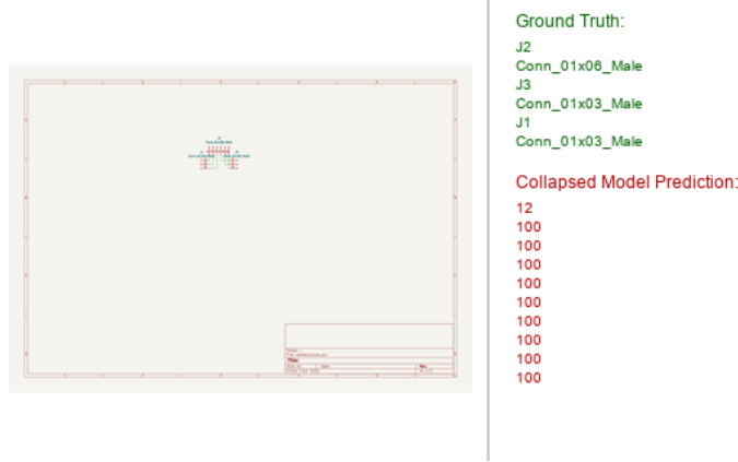
图 4: 旧模型 (V4, +Projector LoRA r = 16 ) 输出: 全部 50 个测试样本输出完全相同的 “12 100 100...”, 多样性 4%, 典型的模态塌缩。
