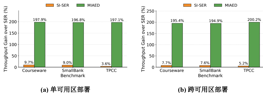
图 6-3 不同部署方式下各策略相对 SER 的吞吐提升百分比
