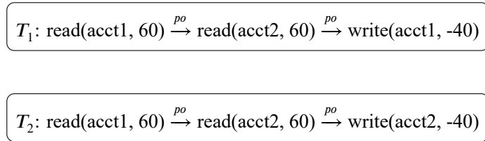
图 2-6 写偏斜示例
