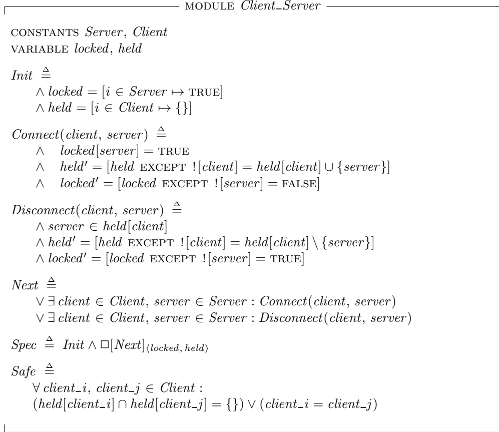
图 2-8 Client_Server 规约
